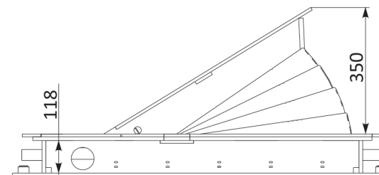
Погружной тип установки
