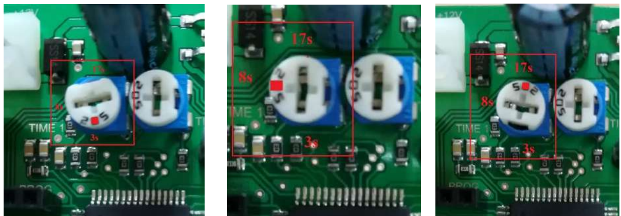
Рис.4 - Регулятор таймаута поднятия и опускания TIME1 в положении 3сек, 8сек, 17сек.
