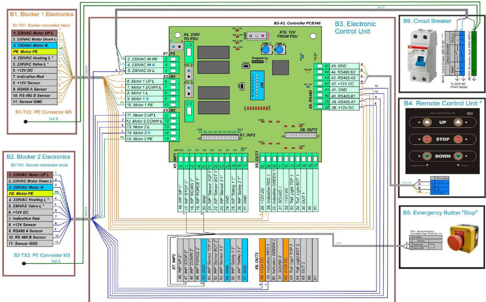
Приложение 2. Схема подключения двух Speedbump или Суслоре RB357, RB358, RB319-1 с встроенной 1-фазной минигидростанцией к блоку управления RB121-2 и дополнительным устройствам.
