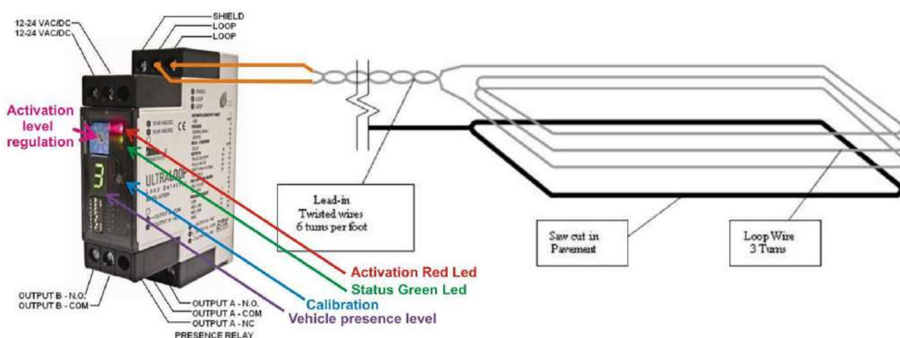
Рис. 12 - Схема подключения индукционной петли к контроллеру индукционной петли блока управления Safety Loop Detector EMX ULTRADIN .
