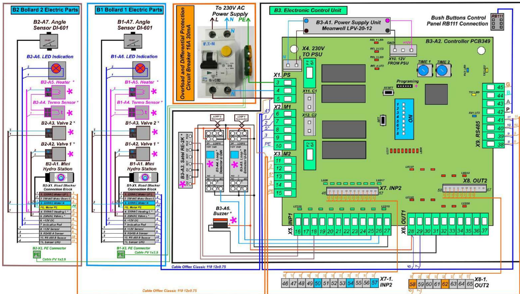
Приложения 2.2. Схема электрическая принципиальная 2-х блокираторов RB357, RB358, RB319-1 с встроенной 1-фазной минигидростанцией, блоком управления RB-121-2 и дополнительными устройствами.
