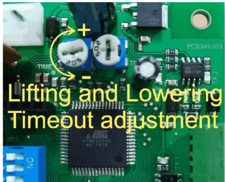
Рис.3 - Регулятор таймаута поднятия и опускания TIME1 .
