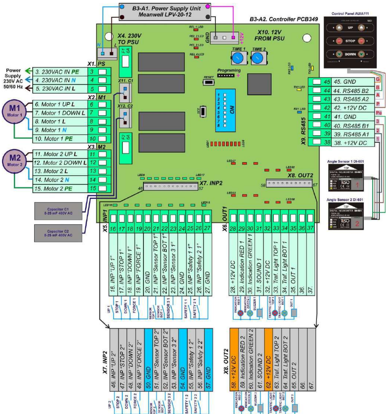
Рис. 2 - Контроллер PCB349 с обозначением его составных частей, выходов и входов.
