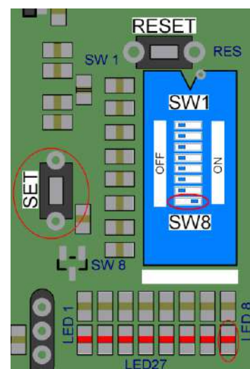
Рис. 6 - Включения калибровки датчика угла DI-601 .
