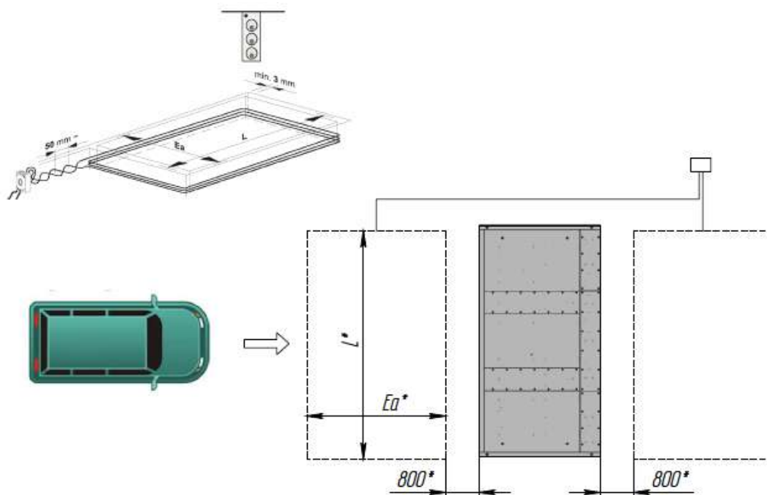
Рис.11 - Пример расположения индукционных петель возле блокиратора.
