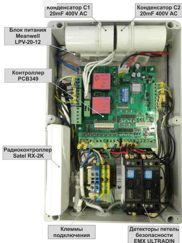
Рис.7 - Блок управления RB121-1/2
